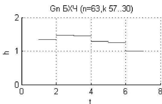
Рисунок 3.8. Нормований показник ефективності кодування (БХЧ n=63 , t= 1, 2, 3, 4, 5, 6 )
