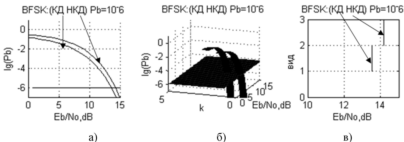
Рисунок 2.15. Енергетична ефективність BFSK(КД), BFSK(НКД) модуляцій: (а) – типові характеристики; (б) - формування УХ; (в) -УХ при P_b=10^{-6}
