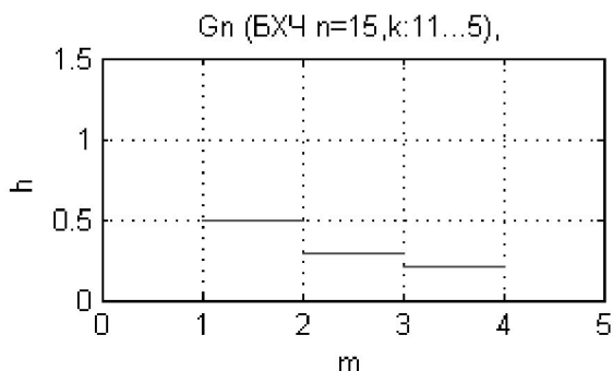
Рисунок 3.10. Нормований показник ефективності кодування (БХЧ n=15 , t=1, 2, 3 )
