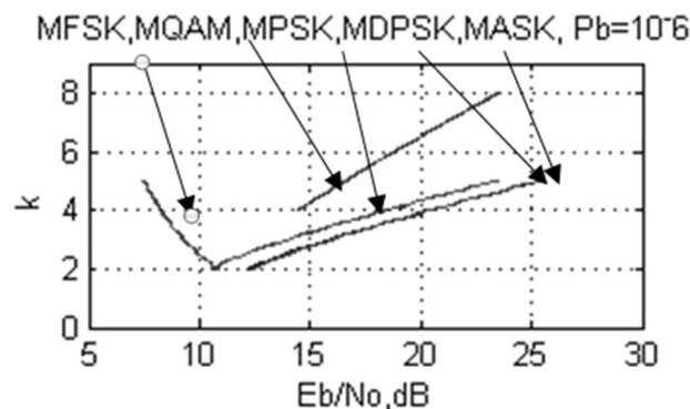
Рисунок 2.14. Порівняння узагальнених характеристик енергетичної ефективності M -мірних модуляцій (MPSK, MDPSK, MASK, MQAM, MFSK)
