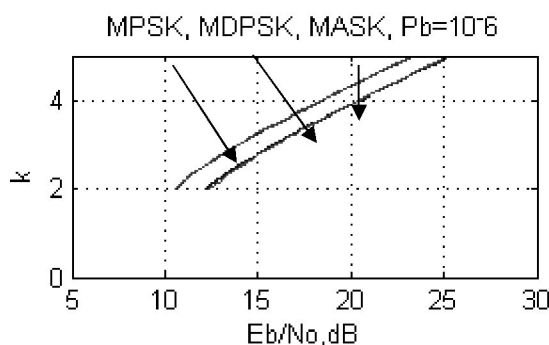
Рисуюнок 2.10. Порівняння узагальнених характеристик енергетичної ефективності M-мірних модуляцій ( MPSK, MDPSK, MASK)
