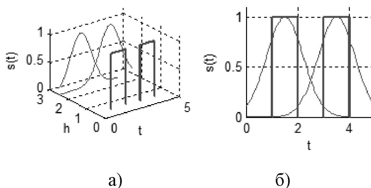
Рисунок 1.5. Проходження цифрового сигналу через ФНЧ: (а)- просторові залежності; (б)- залежності на площині
