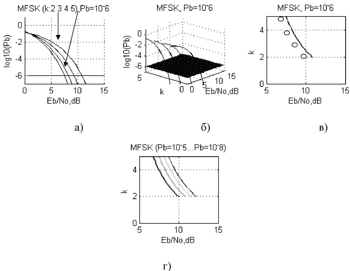
Рисунок 2.13. Енергетична ефективність MFSK модуляції ( відношенні E_b/N_0 – в дБ): (а) - типові характеристики; (б) - формування УХ; (в) - УХ; г) - сімейство УХ
