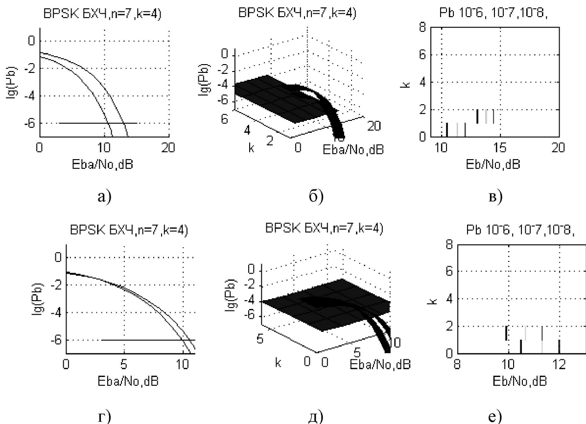
Рисунок 3.11. Залежність P_b для BPSK модуляції при використанні кодів БХЧ ( n=7 ; k(t) 4(1) ): (а), (б), (в) - перший етап, ймовірність P_{bk} (рис.3.3,б), без врахування декодування; (г), (д), (е) - другий етап, ймовірність P_d(P_{bk}) (рис.3.3,в), з врахуванням декодування
