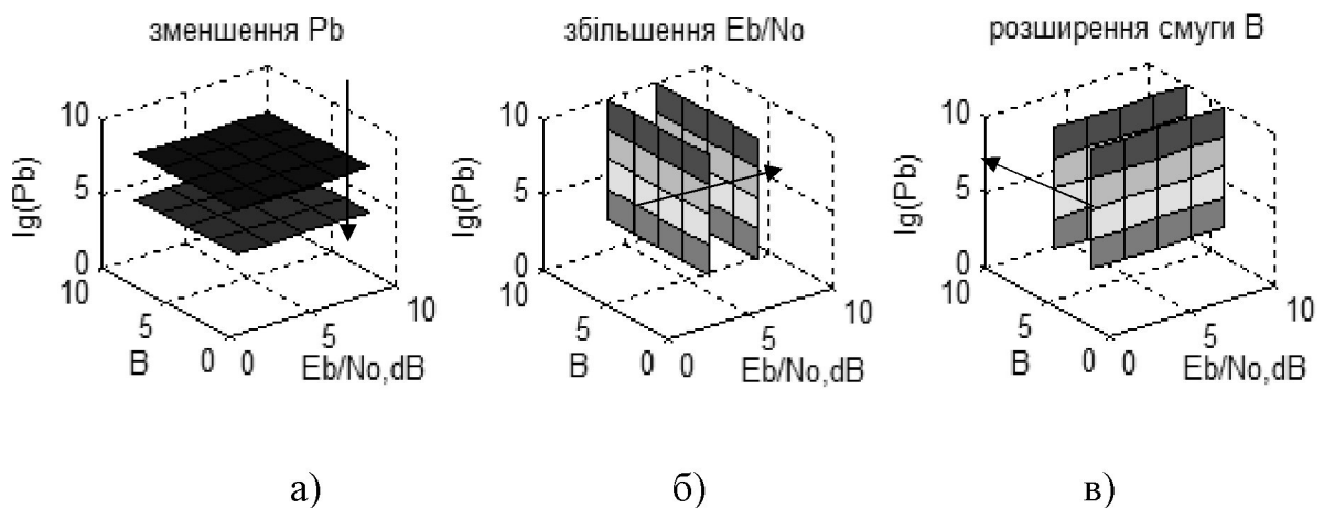
Рисунок 3.1. Шляхи забезпечення необхідного значення P_b \leq (P_b)_{\text{ном}}
