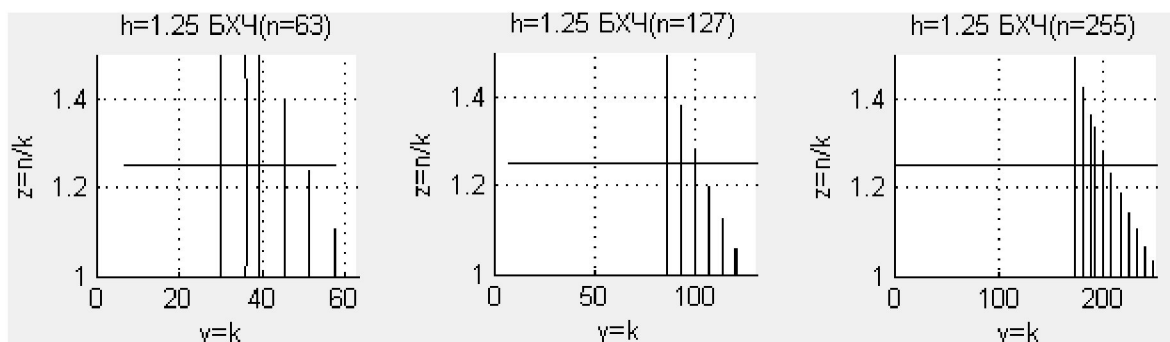
Рисунок 3.4. Вибір кодів БХЧ та можливих компромісів щодо смуги пропускання
