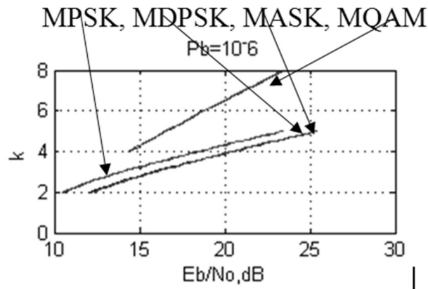
Рисунок 2.12. Порівняння узагальнених характеристик енергетичної ефективності M-мірних модуляцій (MPSK, MDPSK, MASK, MQAM)
