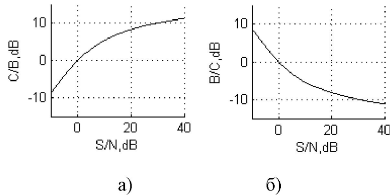
Рисунок 1.7. Залежність від відношення сигнал/шум: (а) - нормованої (C/B) пропускної здатності; (б) - нормованої (B/C) смуги пропускання
