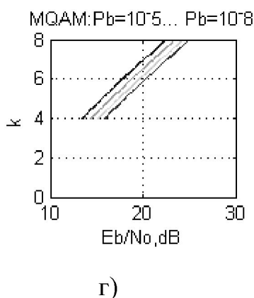
Продовження Рисунок 2.11. Енергетична ефективність MQAM модуляції (відношенні E_b/N_0 – в дБ): (а) - типові характеристики; (б) - формування УХ; (в) - УХ; (г) - сімейство УХ
