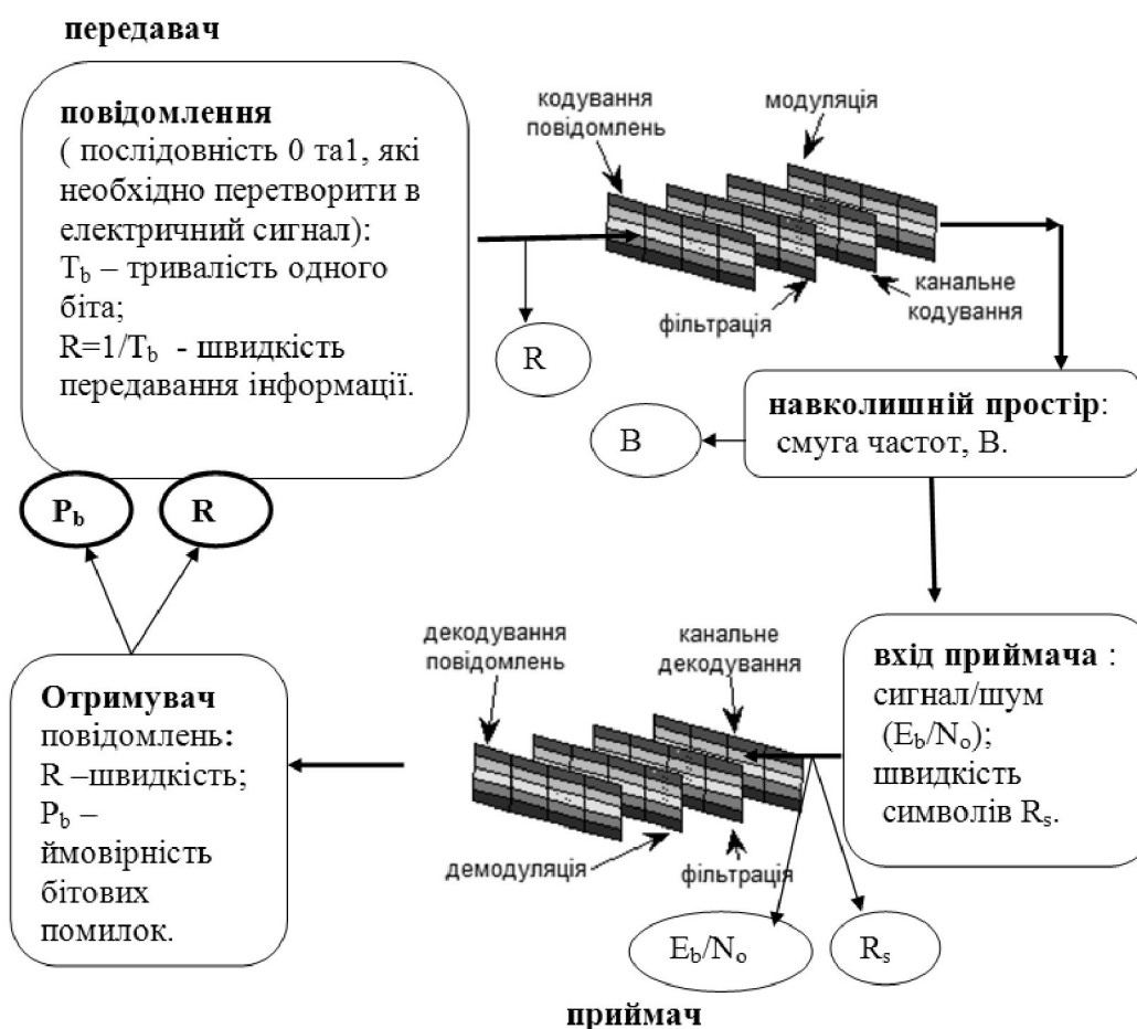
Рисунок 1.3. Типова структурна схема системи безпроводового зв'язку та її основні показники
