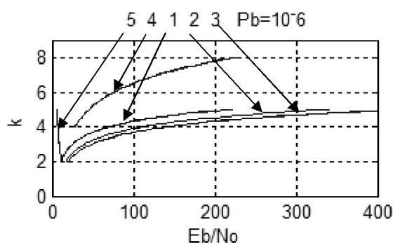
Рисунок 2.17. Необхідні значення відношення сигнал/шум ( E_b/N_0 ) для M-рівневих модуляцій (табл.2.6) при P_b=10^{-6}
