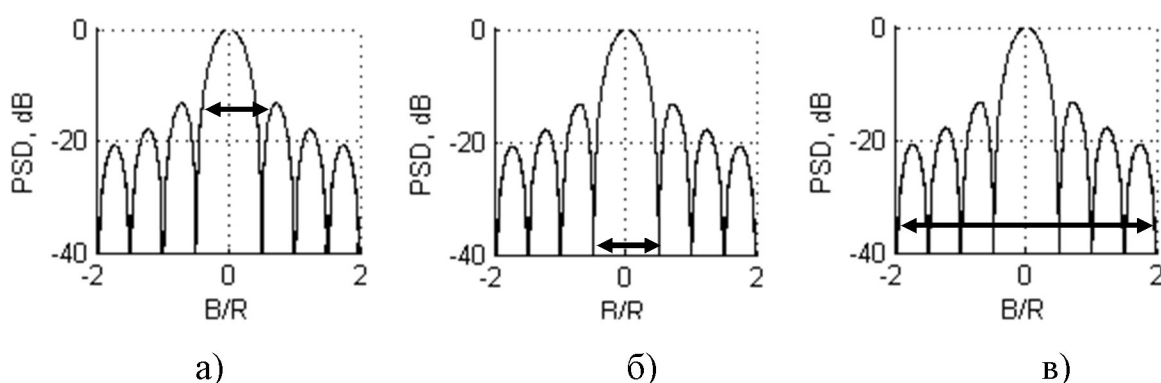
Рисунок 2.18. Ширина смуги цифрових даних: а) половинна потужність; б) за першими нулями; в) 99% потужності
