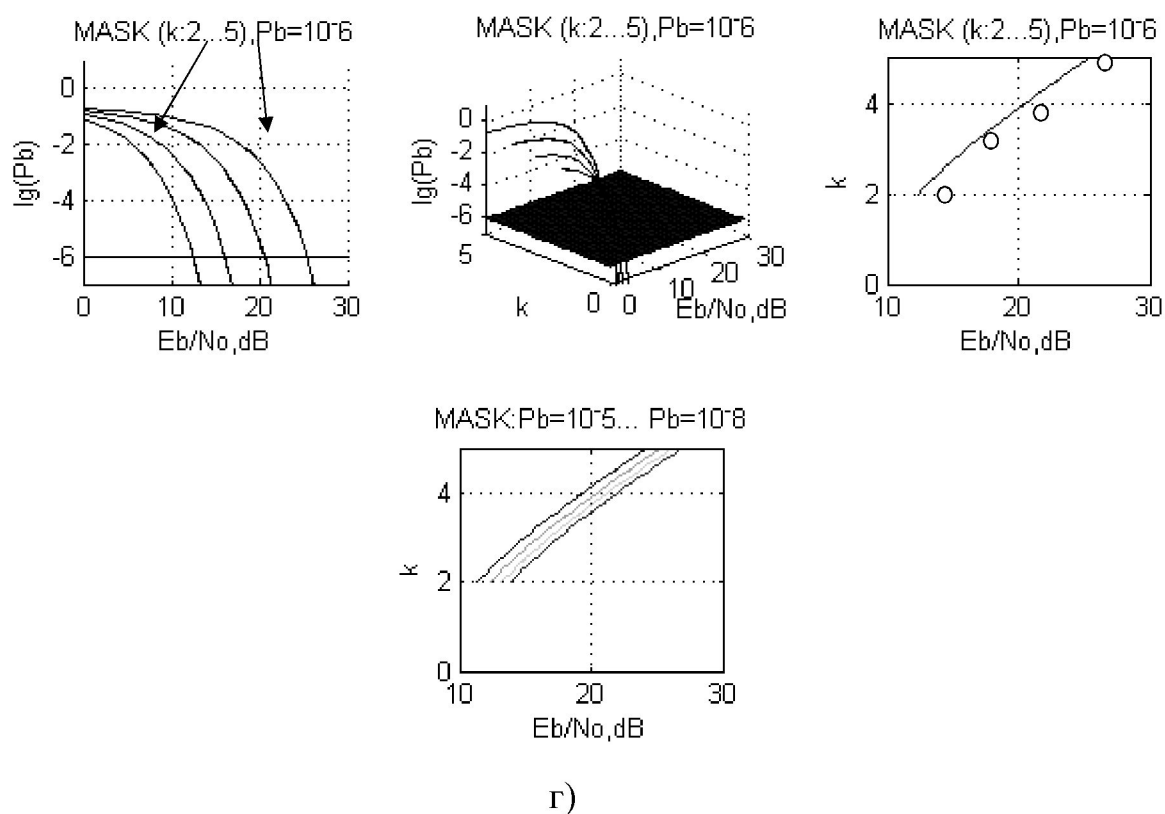
Рисунок 2.9. Енергетична ефективність для MASK модуляції (відношення E_b/N_0 – в дБ): (а) - типові характеристики; (б) - формування УХ; (в) - УХ; г) - сімейство УХ
