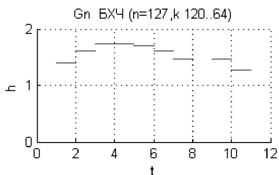
Рисунок 3.9 – Нормований показник ефективності кодування (БХЧ n=127 , t=1, 2, 3, 4, 5, 6, 7, 9, 10 )
