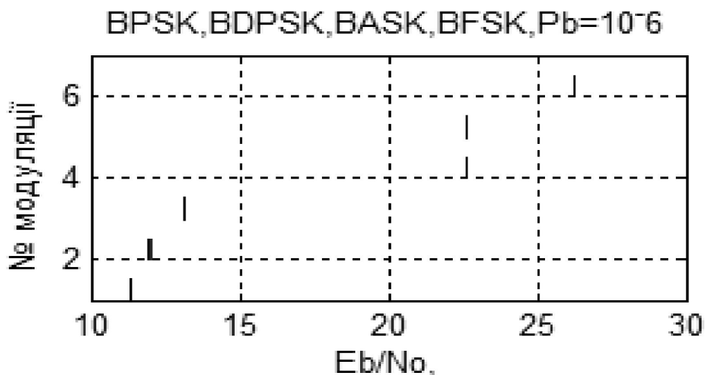
Рисунок 2.16. Необхідні значення відношення сигнал/шум ( E_b/N_0 ) для бінарних модуляцій (табл. 2.5) при P_b=10^{-6}
