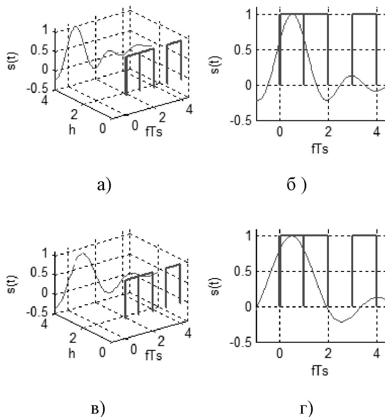
Рисунок 1.6. Проходження цифрового сигналу через ФНЧ: (а, б) - вхідні сигнали та вихідний сигнал 1-го імпульсу при V=1/2T_s ; (в, г) - вхідні сигнали та вихідний сигнал 1-го імпульсу при V<1/2T_s
