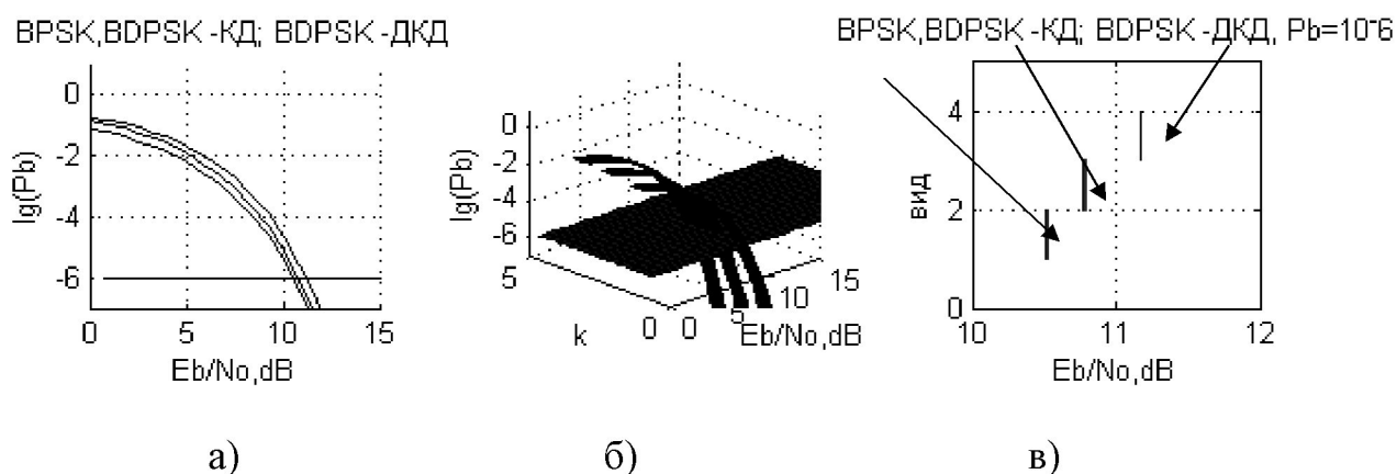
Рисунок 2.8. Енергетична ефективність BPSK (КД), BDPSK (КД) та BDPSK (ДКД) модуляцій: (а) - типові характеристики; (б) - формування УХ; (в) – УХ
