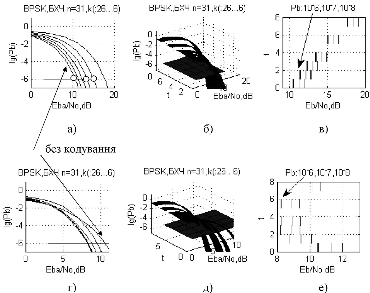
Рисунок 3.5. Залежність P_b для BPSK модуляції при використанні кодів БХЧ ( n=31 ; k(t) 26(1), 21(2), 16(3), 11 (5), 6(7): (а), (б), (в) - перший етап, ймовірність P_{bk} (рис.3.3,б), без врахування декодування; (г), (д), (е) другий етап – ймовірність P_d(P_{bk}) (рис.3.3,в), з врахуванням декодування
