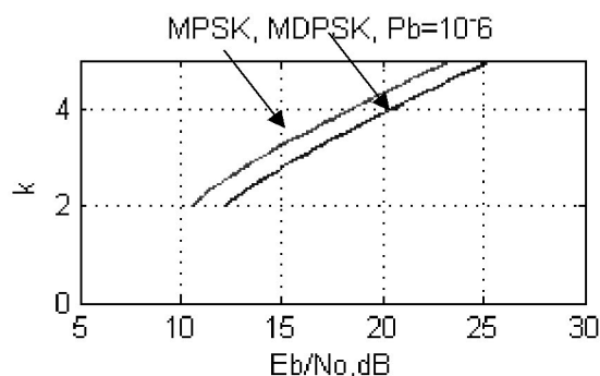
Рисунок 2.7. Порівняння енергетичної ефективності MPSK та MDPSK модуляцій
