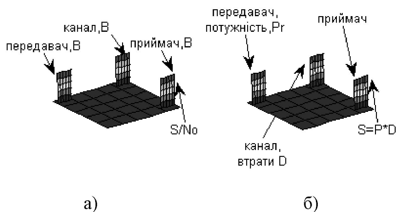
Рисунок 1.2. Ресурси системи безпроводового зв'язку: (а) – необхідні ресурси; (б) – формування ресурсів
