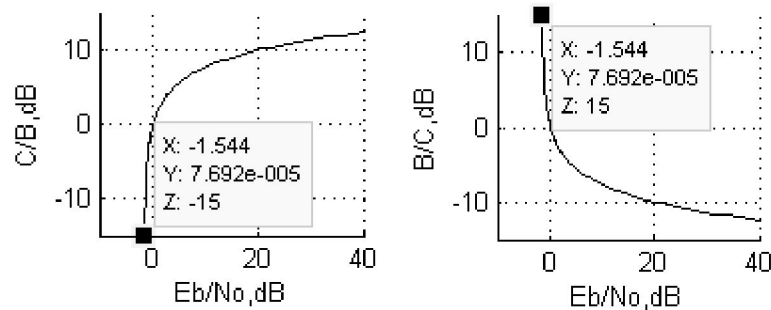
Рисунок 1.8. Залежність нормованої пропускної здатності ( C/V ) та нормованої смуги пропускання ( V/C ) каналу від відношення E_b/N_o
