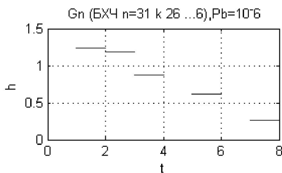
Рисунок 3.6. Нормований показник ефективності кодування (БХЧ n=31 , t= 1, 2, 3, 5, 7 )
