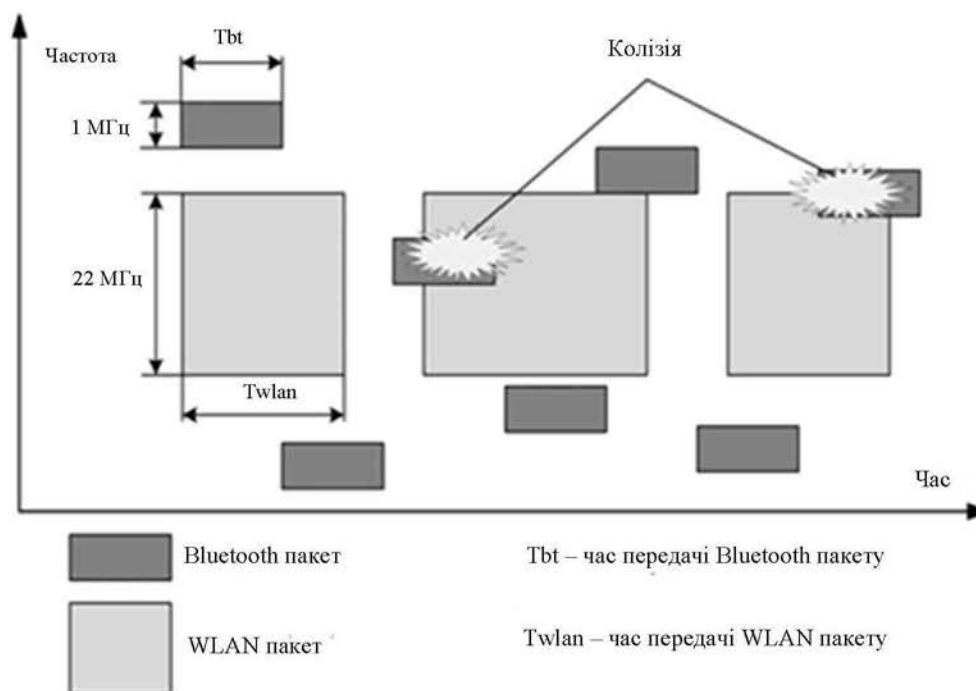
Рисунок 1.4. Приклад зіткнення пакетів Wi-Fi і Bluetooth
