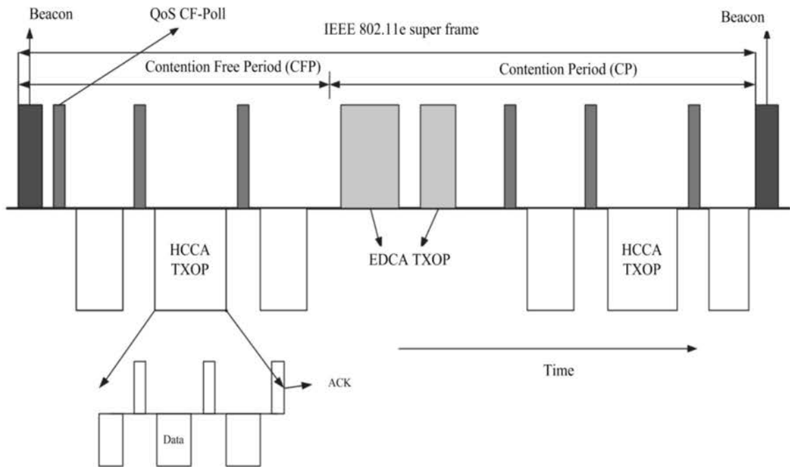
Рисунок 2.4. Робота IEEE 802.11 e HCCA в суперкадрі
