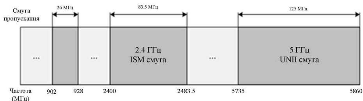
Рисунок 1.1. ISM-смуга
