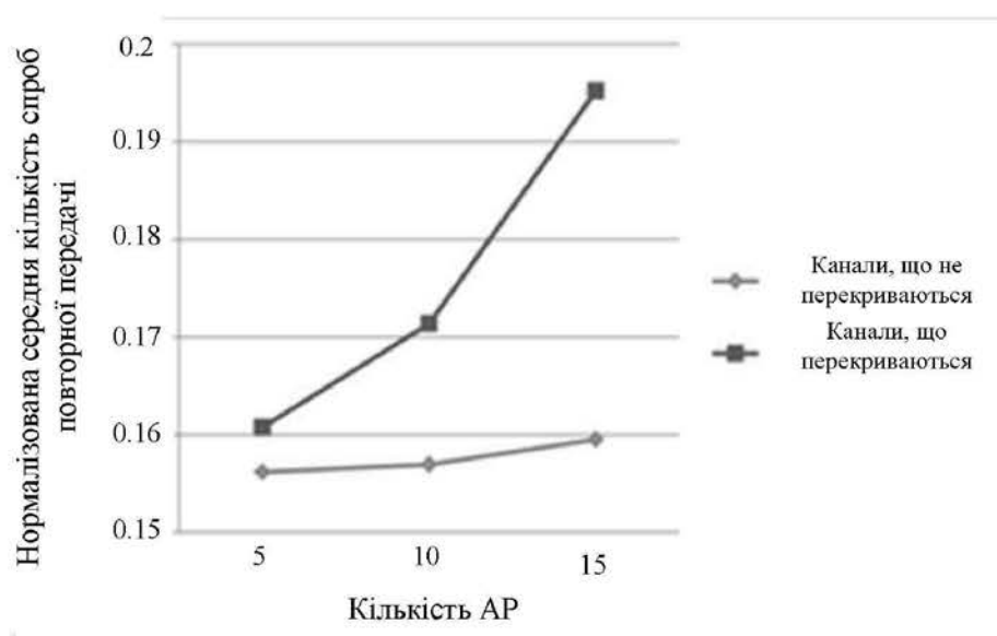
Рисунок 1.13. Вплив перекриваються каналів з точки зору кількості спроб повторної передачі
