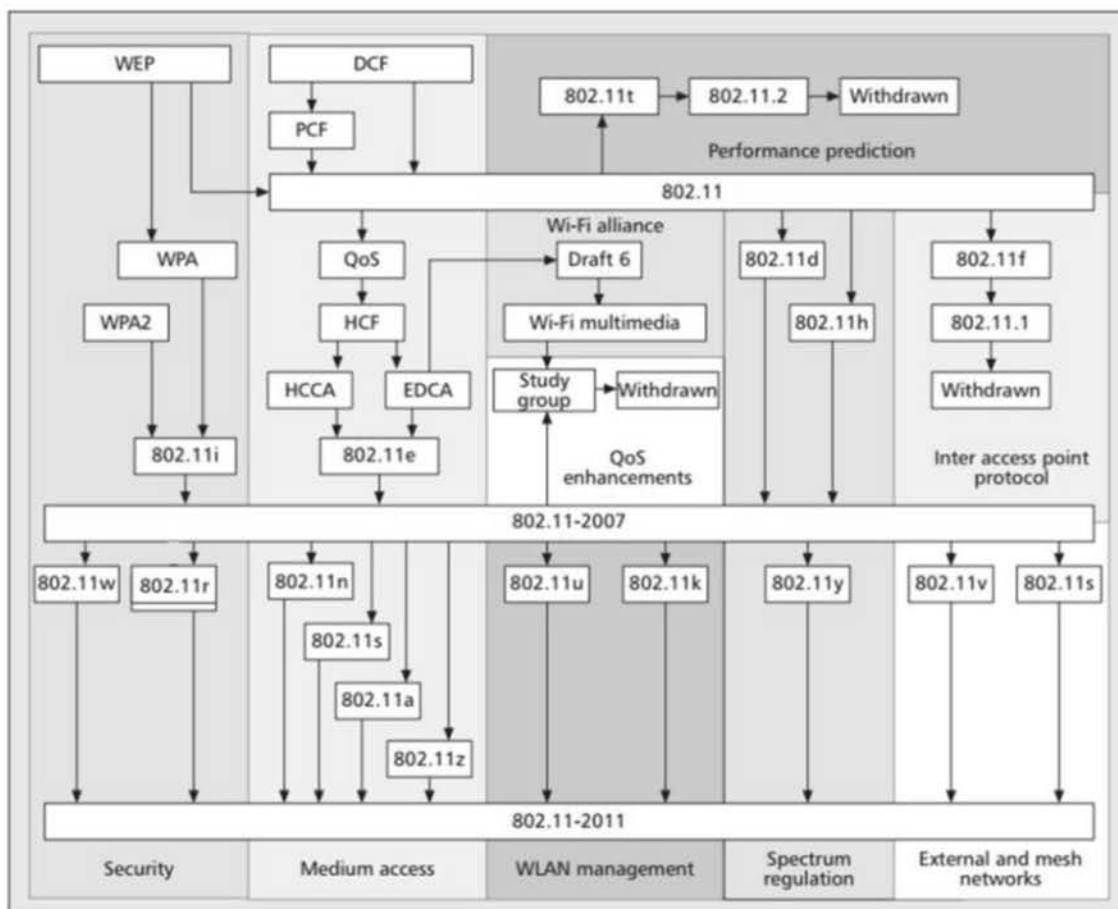
Рисунок 1.3. Поправки IEEE 802.11 MAC-рівня
