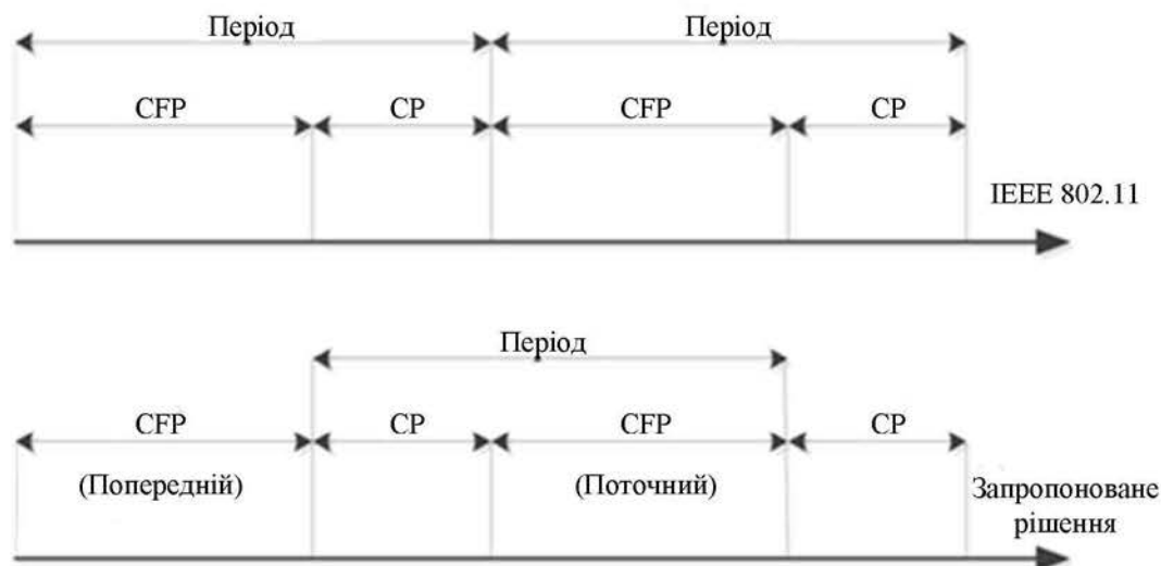
Рисунок 3.10. Концепція «періоду» в запропонованому рішенні
