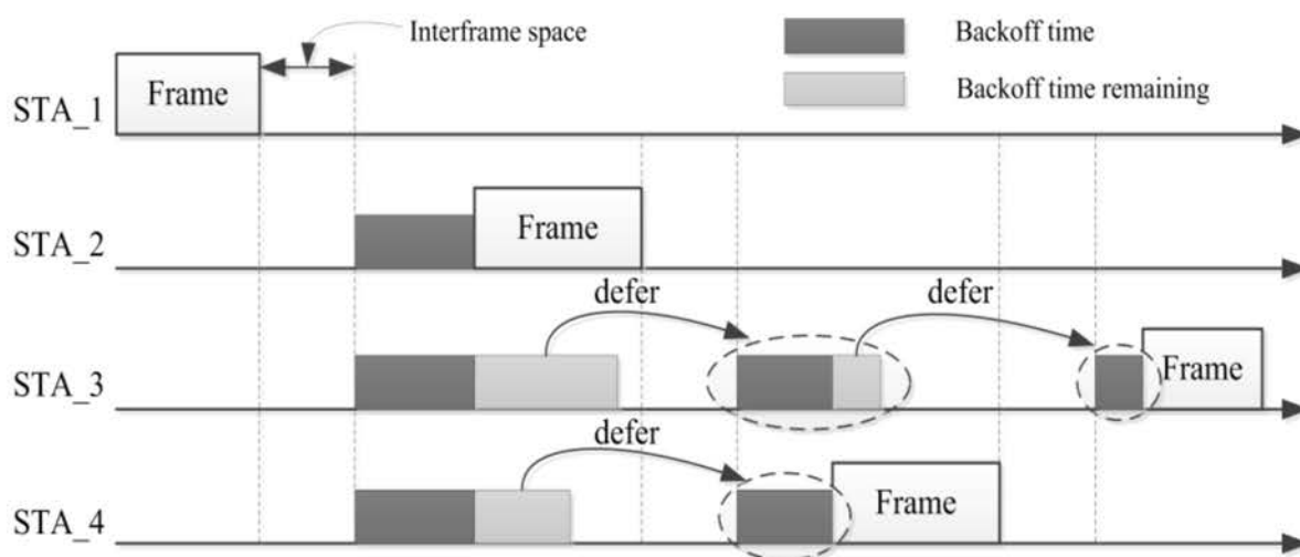
Рисунок 2.1. Принцип роботи механізму конкуренції
