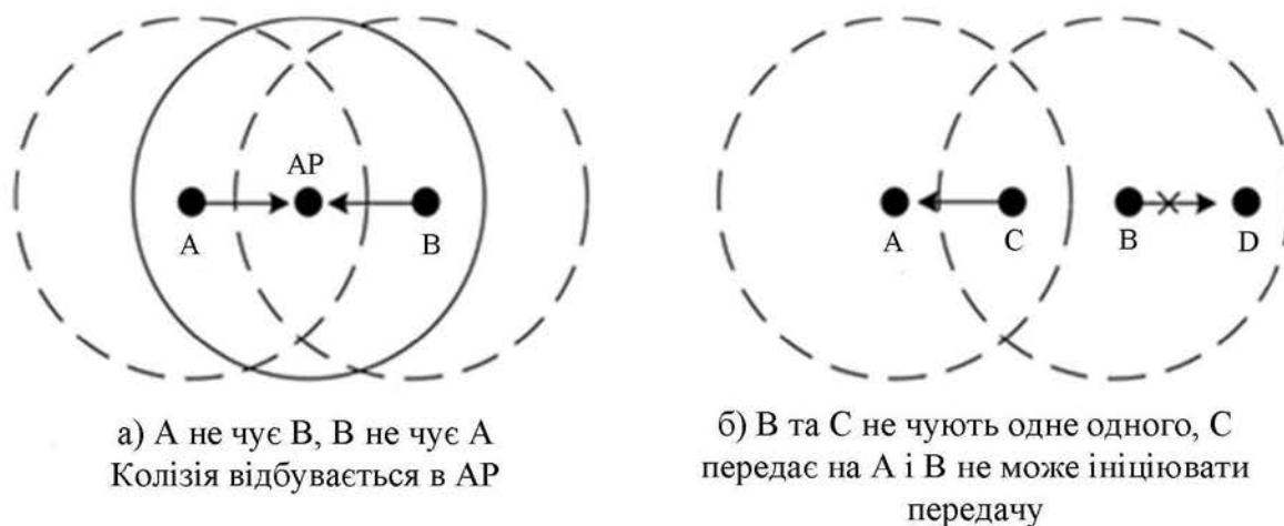
Рисунок 1.7. а) Проблема прихованого вузла б) Проблема незахищеного вузла
