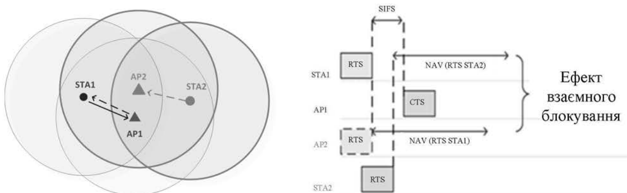
Рисунок 1.10. Ефект взаємного блокування
