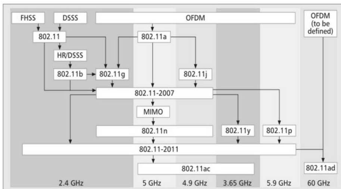
Рисунок 1.2. Поправки IEEE 802.11 PHY-рівня і їх залежності
